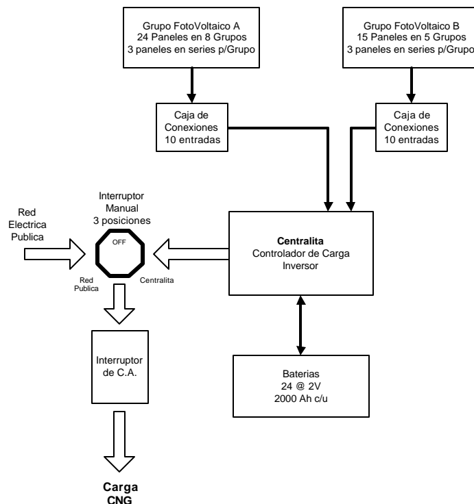
Esquemas del Sistema Fotovoltaico existente en el Colegio Nacional Galapagos
